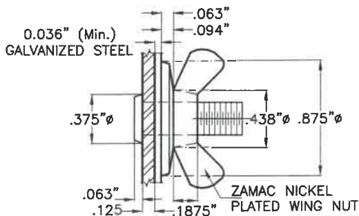
DETAIL 1 SCALE: 1"=1"
