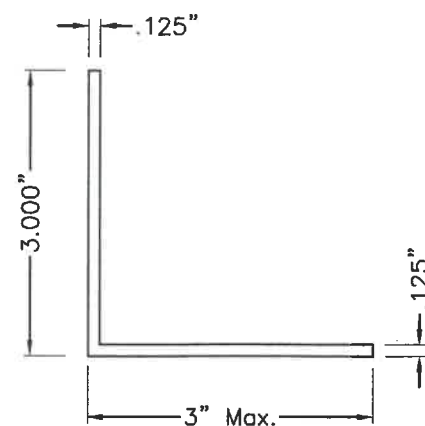
⑦ 3"x3"(Max.) ALUM. ANGLE
