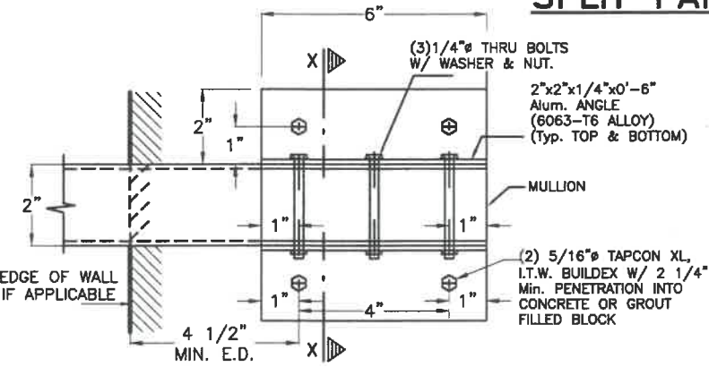
ELEVATION SCALE: 1/4" = 1"
