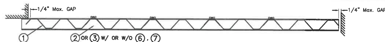
SECTION A-A
